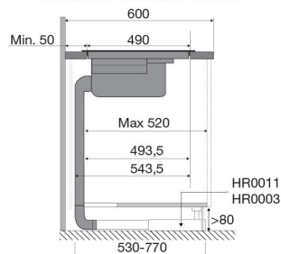
Zijaanzicht werkblad 600 mm Combinatie HR0003 en HR0011
